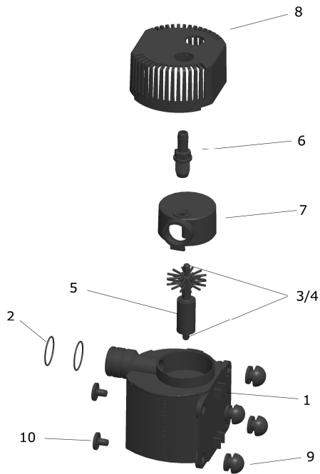
Fig. 2: Pompa Venturi AQ 750 con girante
